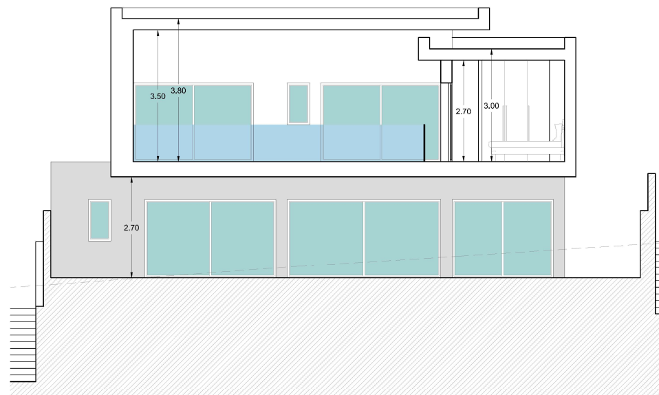
SECCION DD'
