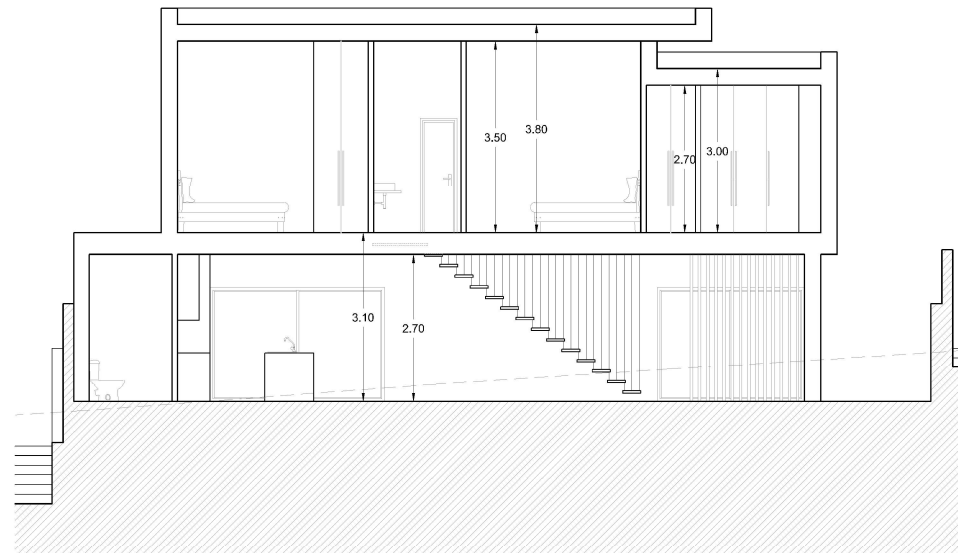
SECCION EE'
