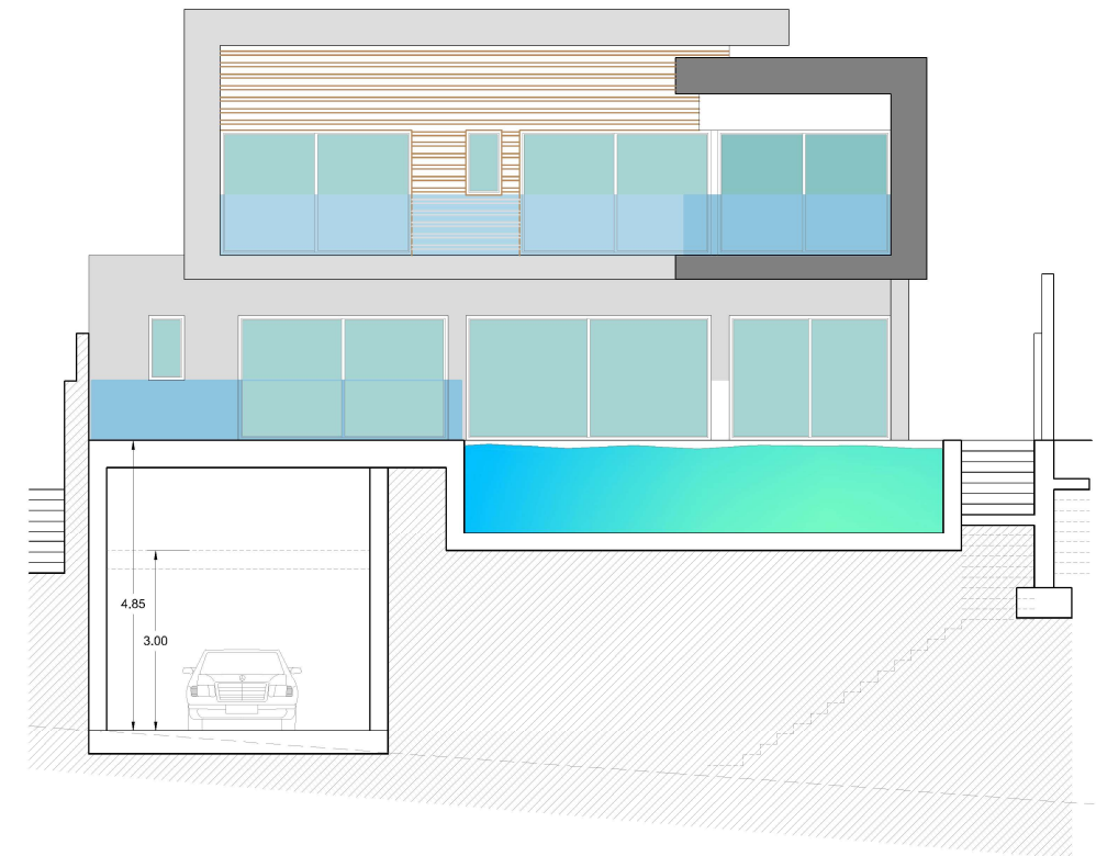
SECCION GG'
