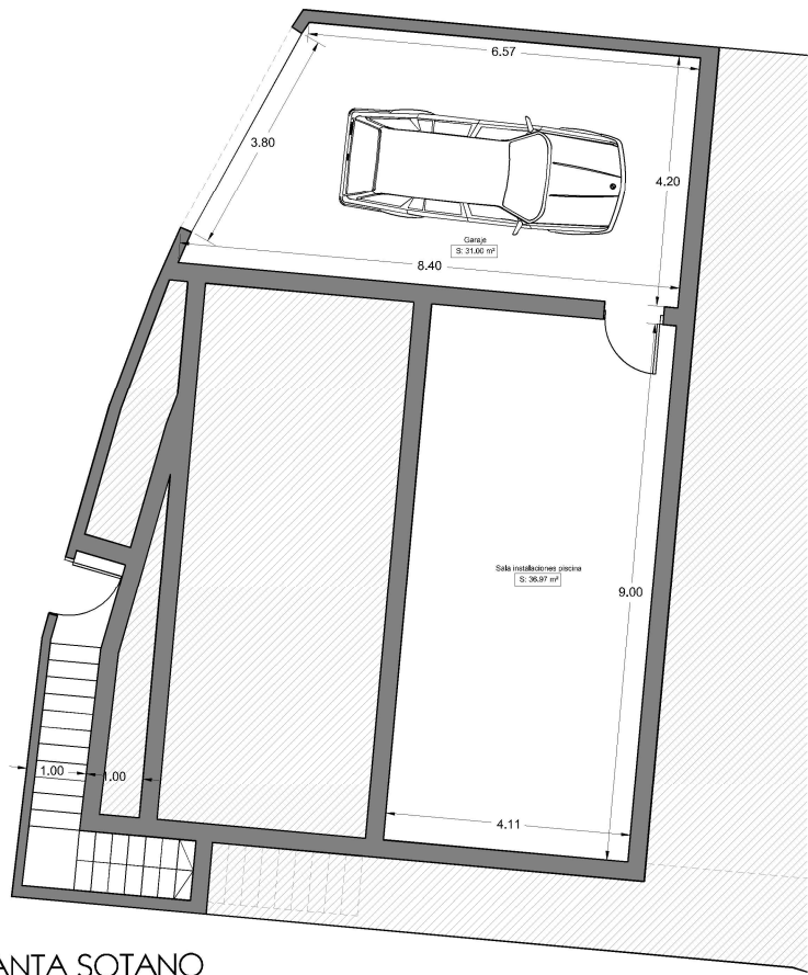
PLANTA SOTANO
