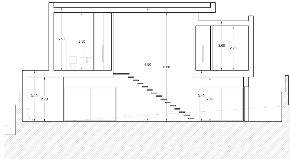
SECCION FF'
