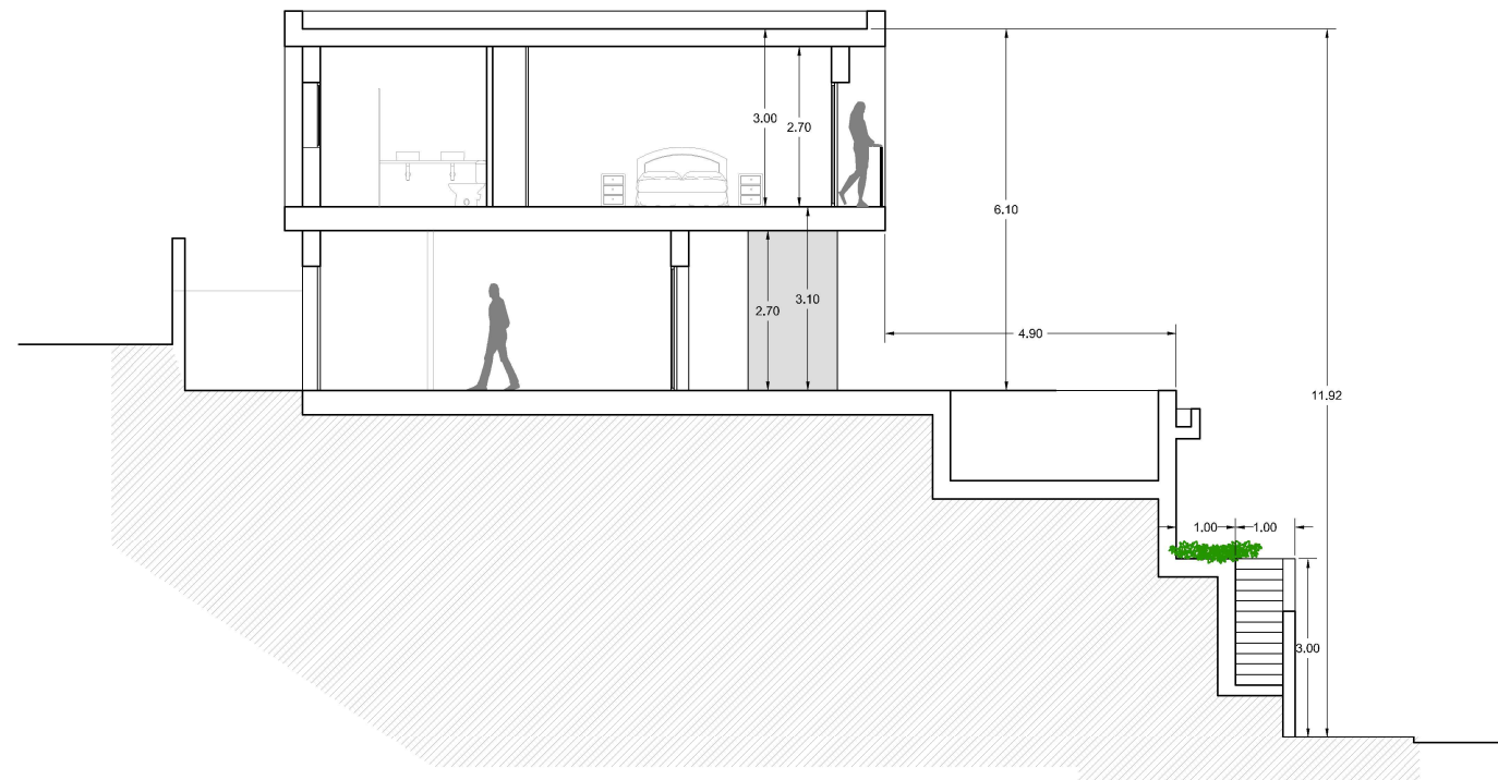
SECCION II'
